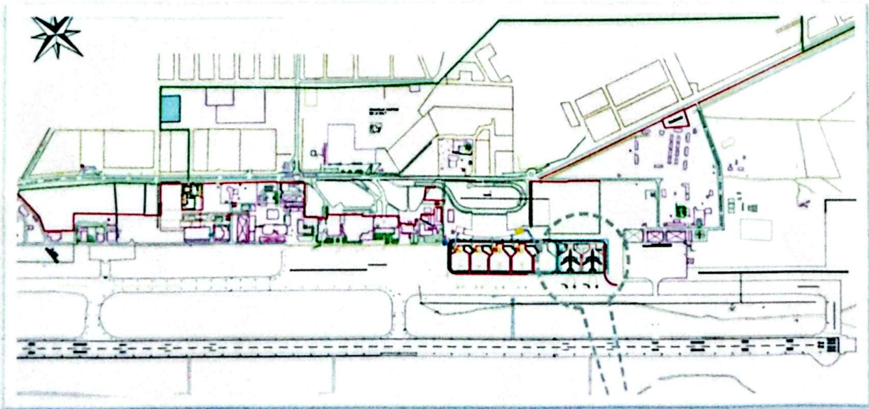
Extrait du plan de l'extension de l'hydrant de Lomé Tonkoin
