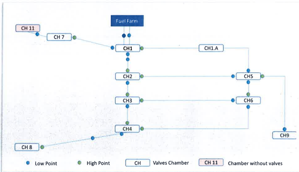
Extrait du schéma de l'hydrant de Beyrouth
