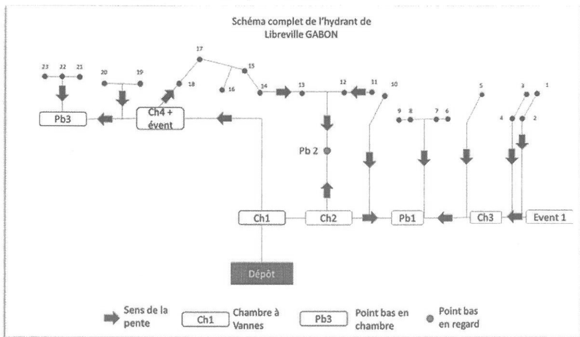
Extrait du schéma de l'hydrant de Libreville
